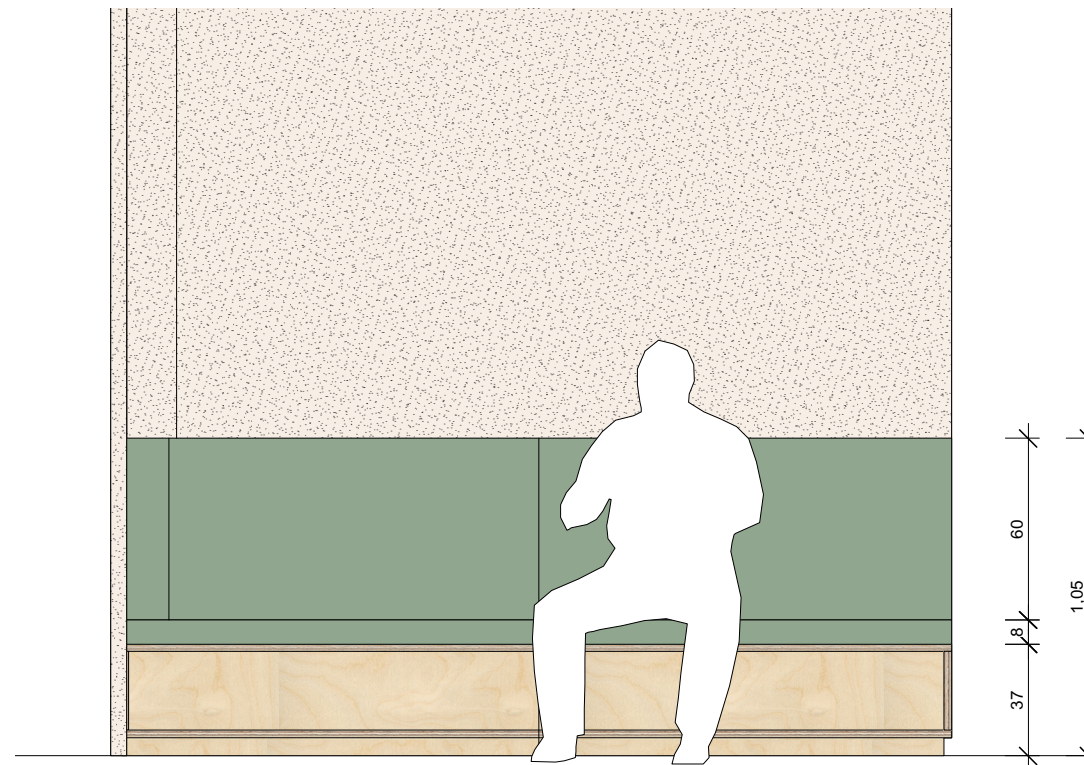
Frontansicht M 1:25
