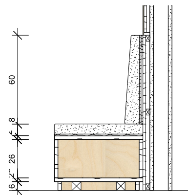
Schnitt A-A M 1:25
