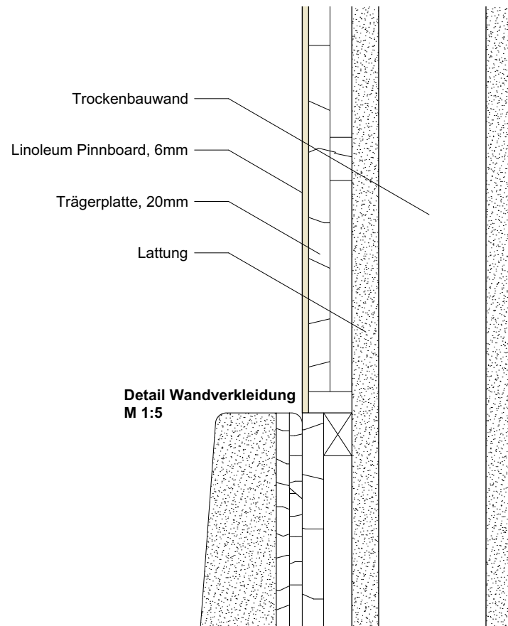
Detail Wandverkleidung M 1:5
